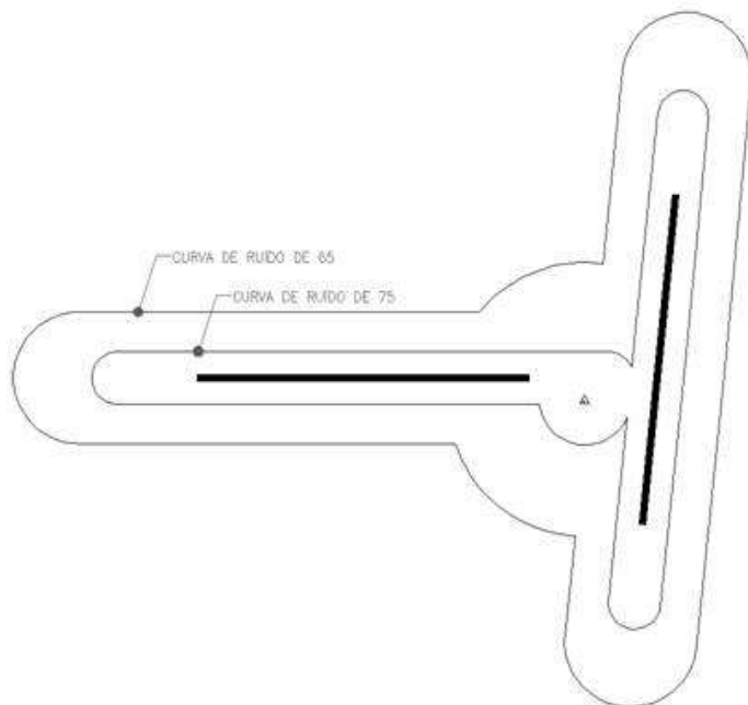
FIGURA C-3- Composição de curvas de ruído para aeródromos com mais de uma pista e FATO. (Redação dada pela Resolução nº 609, de 23.02.2021) (../resolucoes/2021/resolucao-no-609-23-02-2021)
