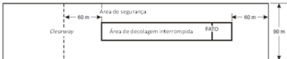
Figura 155.209-3 - Área de segurança para FATO com operação por instrumento
