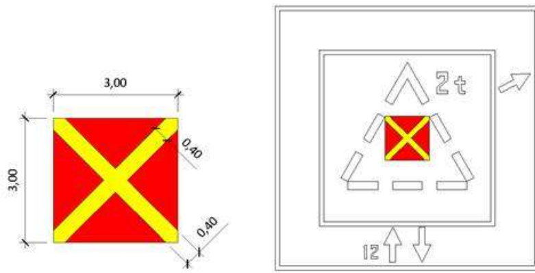
a) Dimensões da sinalização horizontal de interdição de FATO
