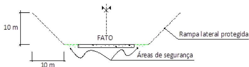
Figura 155.209-2 - Rampa lateral protegida além da área de segurança.
