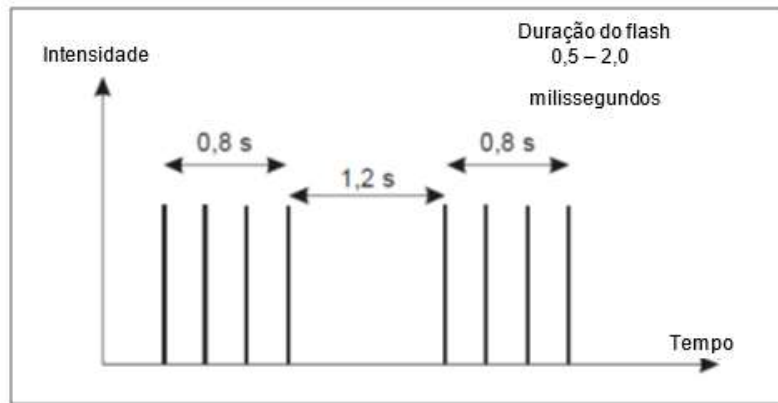
Figura 155.339-1 - Características do flash do Farol de Heliponto
