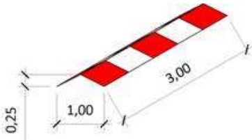
Figura 155.315-2 – Sinalizador de perímetro de FATO tipo pista de pouso e decolagem.
