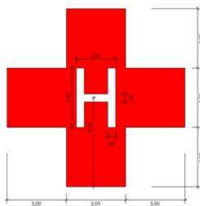
Figura 155.303-2 - Sinalização horizontal de identificação de heliponto em hospital.
