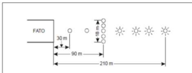
Figura 155.341-1 - Sistema de luzes de aproximação
